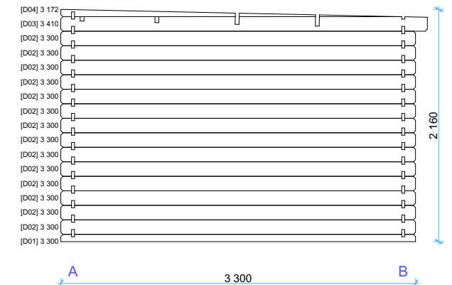
Wall D 1:50
