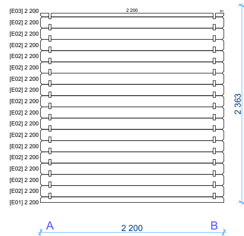
Wall E 1:45
