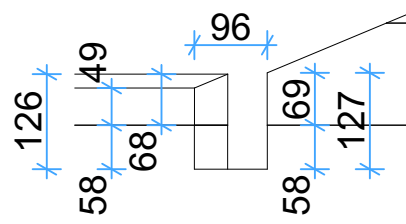
W-02-1 1:10
