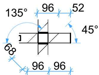
W-01 1:10
