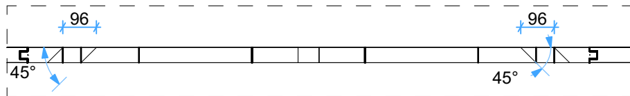
Wall C-1 1:15
