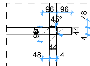
Wall B 1:15
