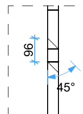
Wall G 1:15
