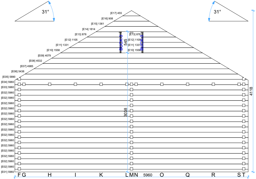
1:50 Wall E
