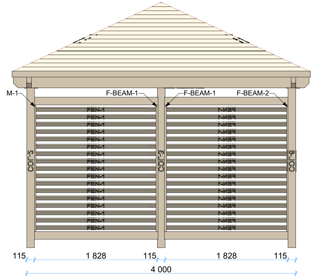
Right Elevation
