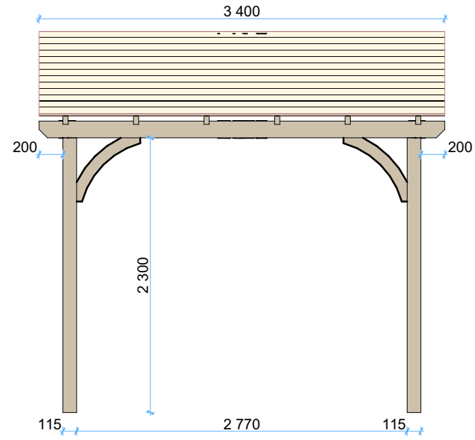
Right Elevation
