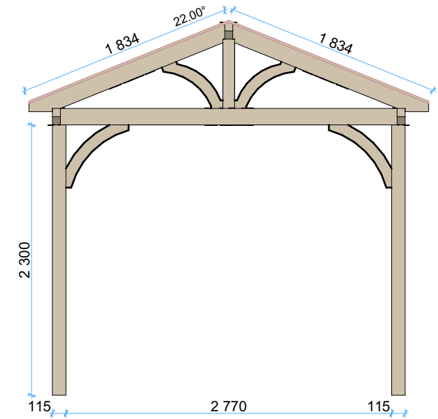
Right Elevation
