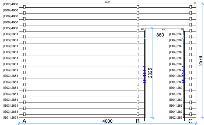
Wall E
