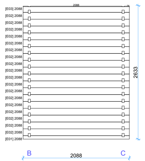
Wall E
